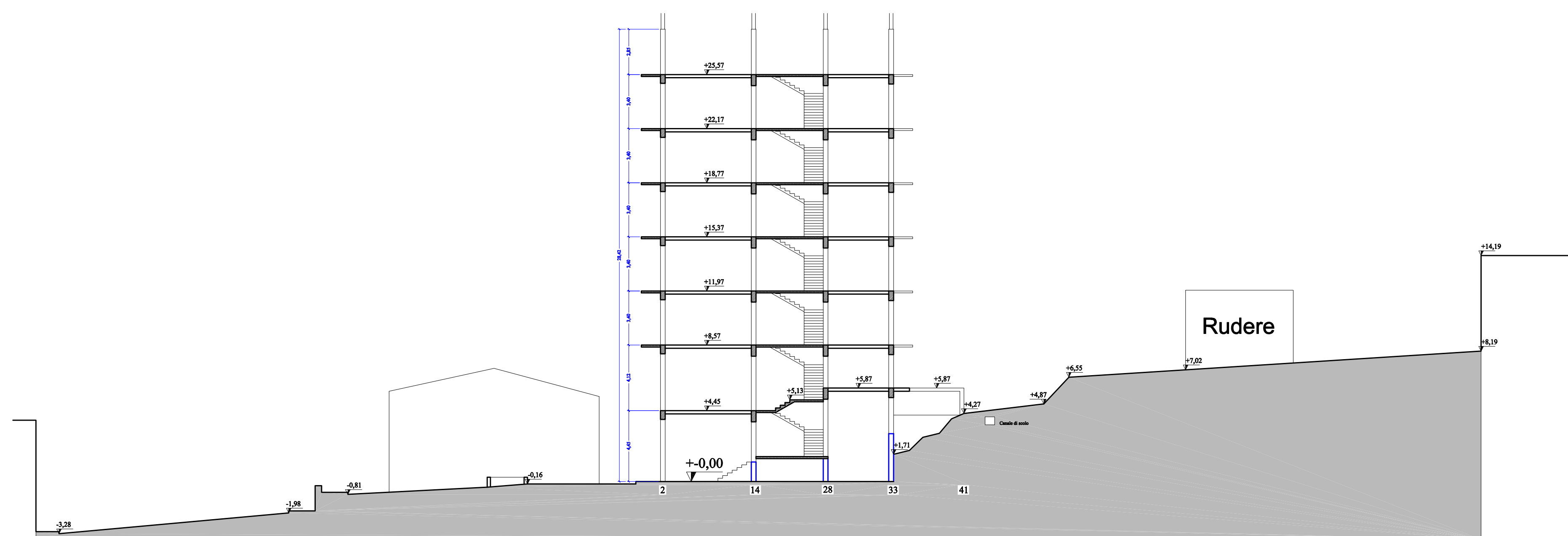
Sezione A-A
